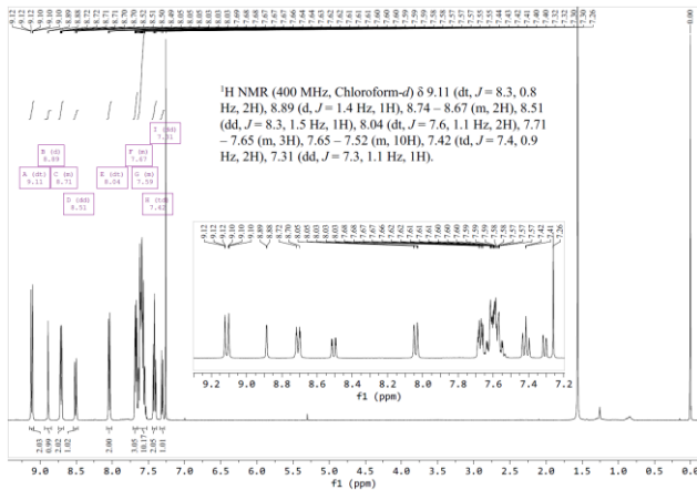
Figure 1. 1 H NMR spectrum of PCPF-TRz
